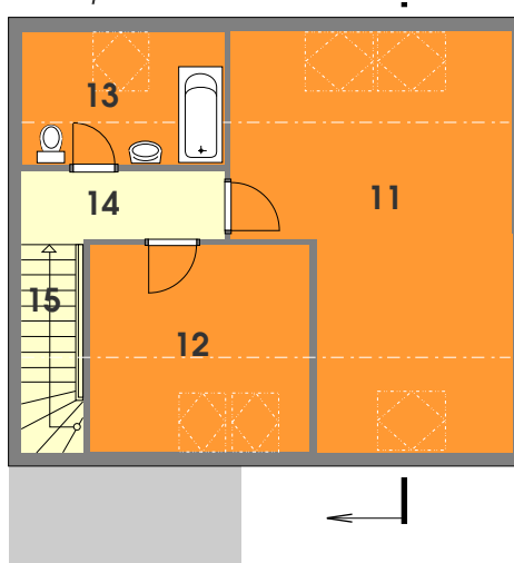
Мансарда
